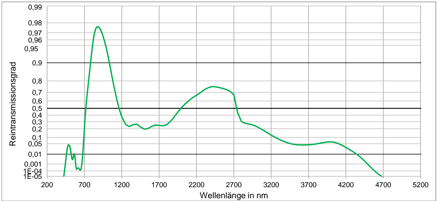
Reintransmissionsgrad t_i bei der Referenzdicke Die Reintransmissionsgrade, tabellarisch und graphisch, sind als Richtwerte zu verstehen.
