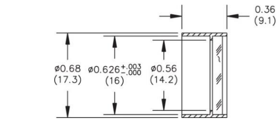
A08087 Input Lens Diffuser (Opal)
