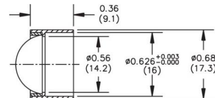
A08086 Input Lens Diffuser
