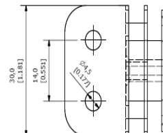
Ángulos de montaje
