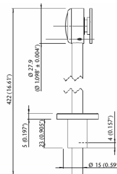
Postes de montaje, vista lateral
