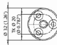
Postes de montaje, capuchón terminal
