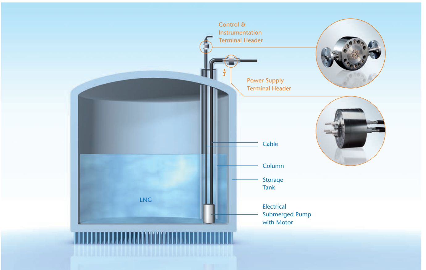
터미널 헤더는 삼상 전원, 계장 및 제어 신호를 LNG 수중 펌프, 터빈 익스팬터, 콤프레서에 공급하는 밀봉 피드스루입니다.
