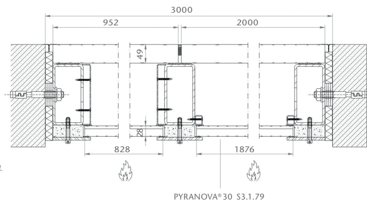
Vista lateral del vidrio pisable ensayado
