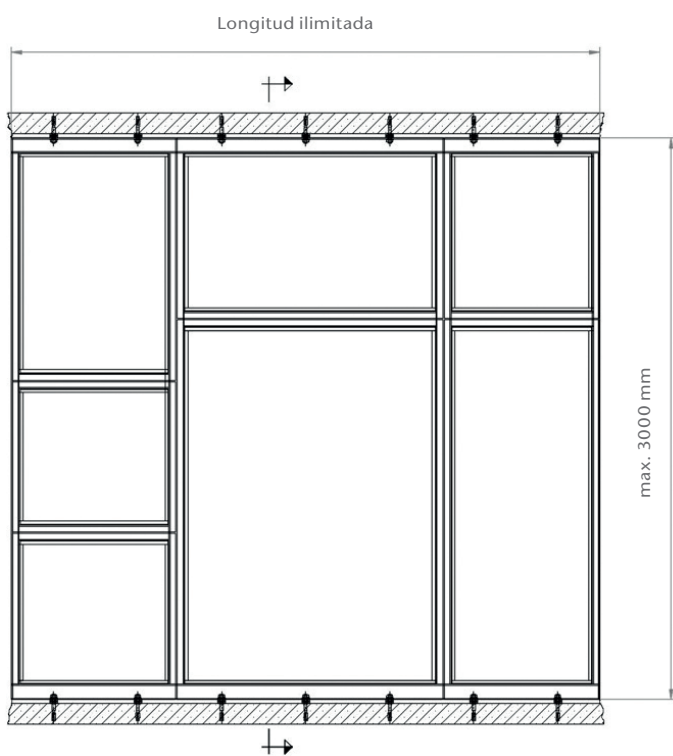
Vista frontal del vidrio pisable ensayado
