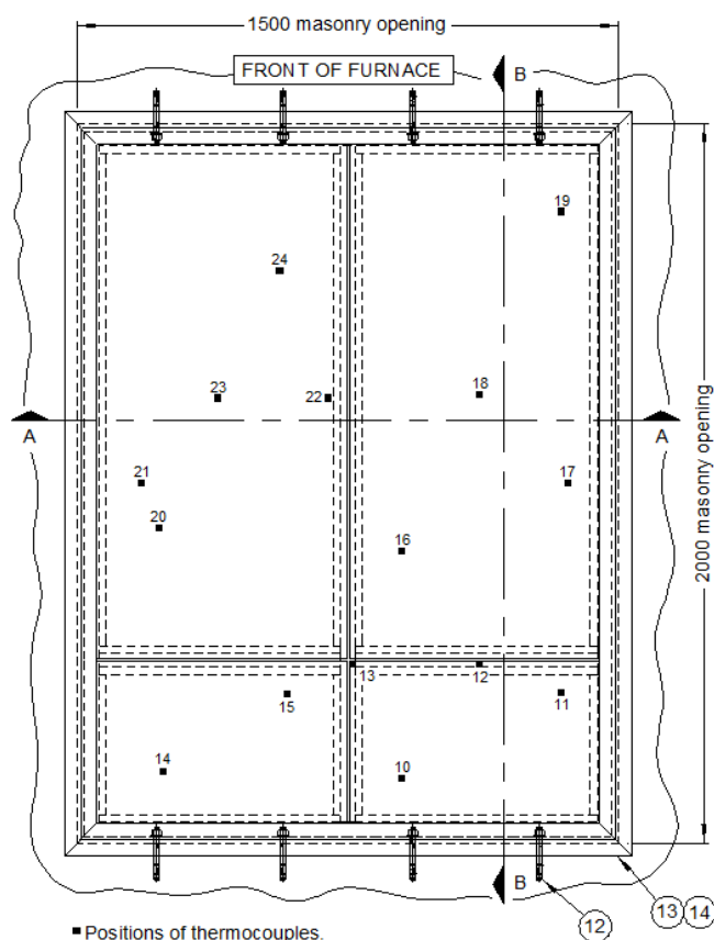
Vista frontal del vidrio pisable ensayado
