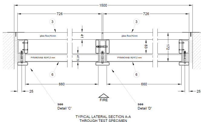
Vista lateral del vidrio pisable ensayado
