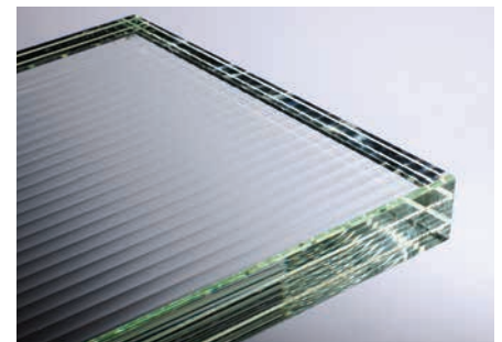
Verbundglas: 8 mm RIVULETTA® mit 1,52 mm PVB Folie, 10 mm Floatglas, 1,52 mm PVB Folie und 8 mm RIVULETTA®
