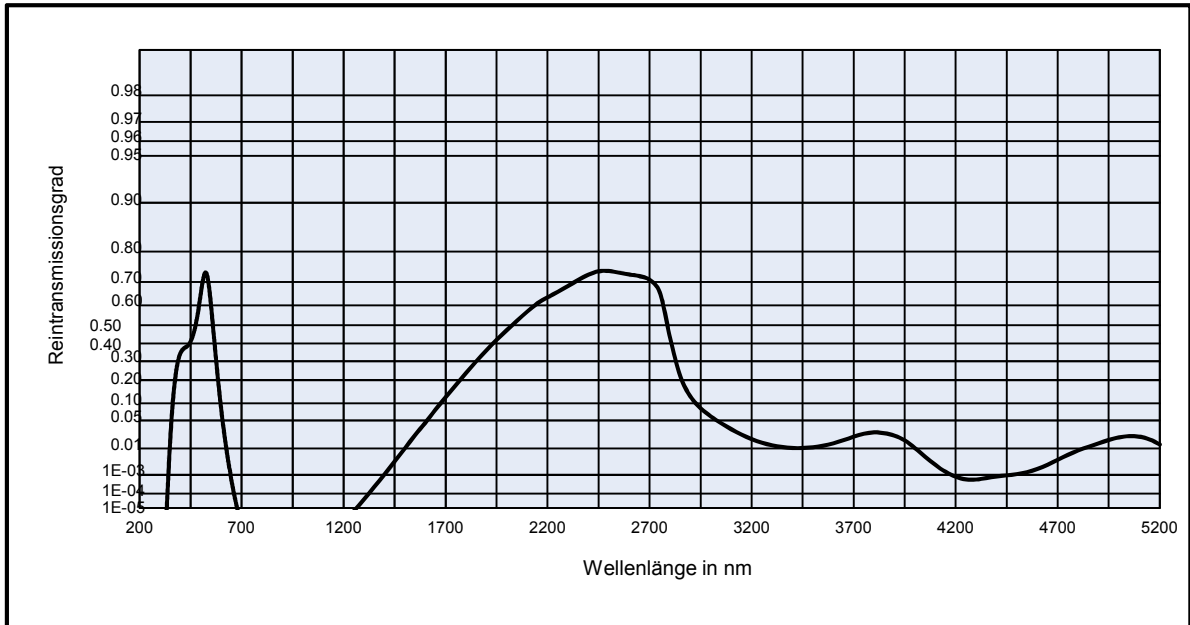
Reintransmissionsgrad t_i bei der Referenzdicke d = 1 \text{ mm} Die Reintransmissionsgrade, tabellarisch und graphisch, sind als Richtwerte zu verstehen.
