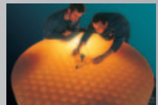
Bei dem „Magellan“-Teleskop kommen auf der Rückseite gewichtserleichterte, ausgefräste „Zerodur“ Leichtgewichts-Spiegelträger zum Einsatz.
